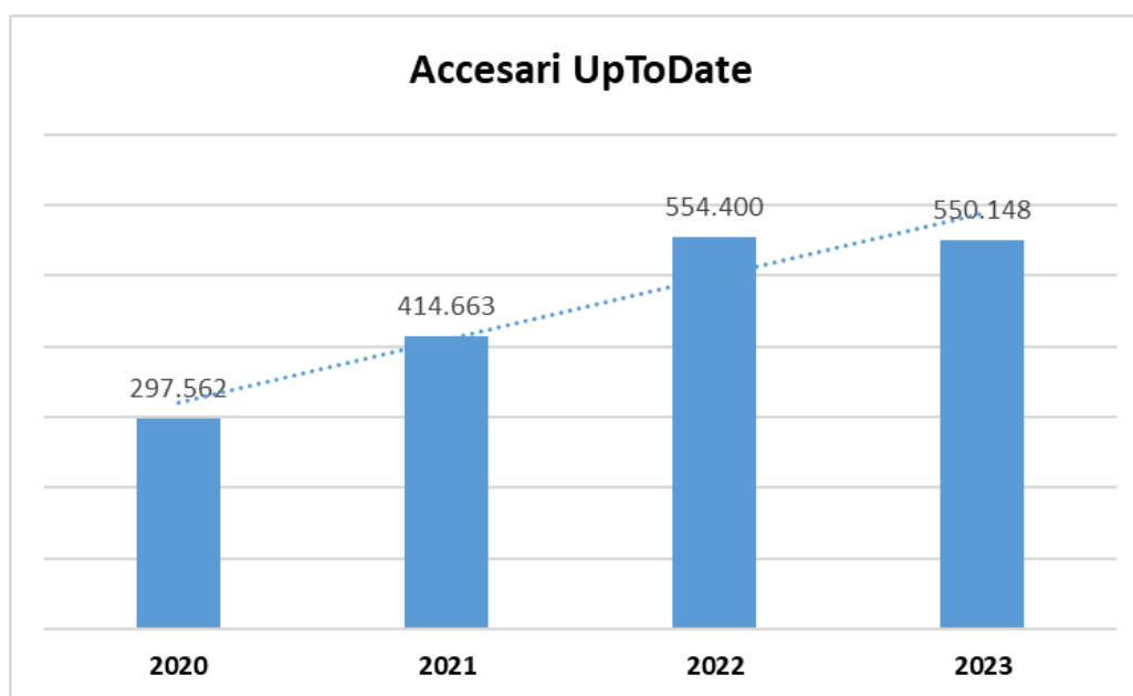
Fig. 4 Accesări UptoDate
